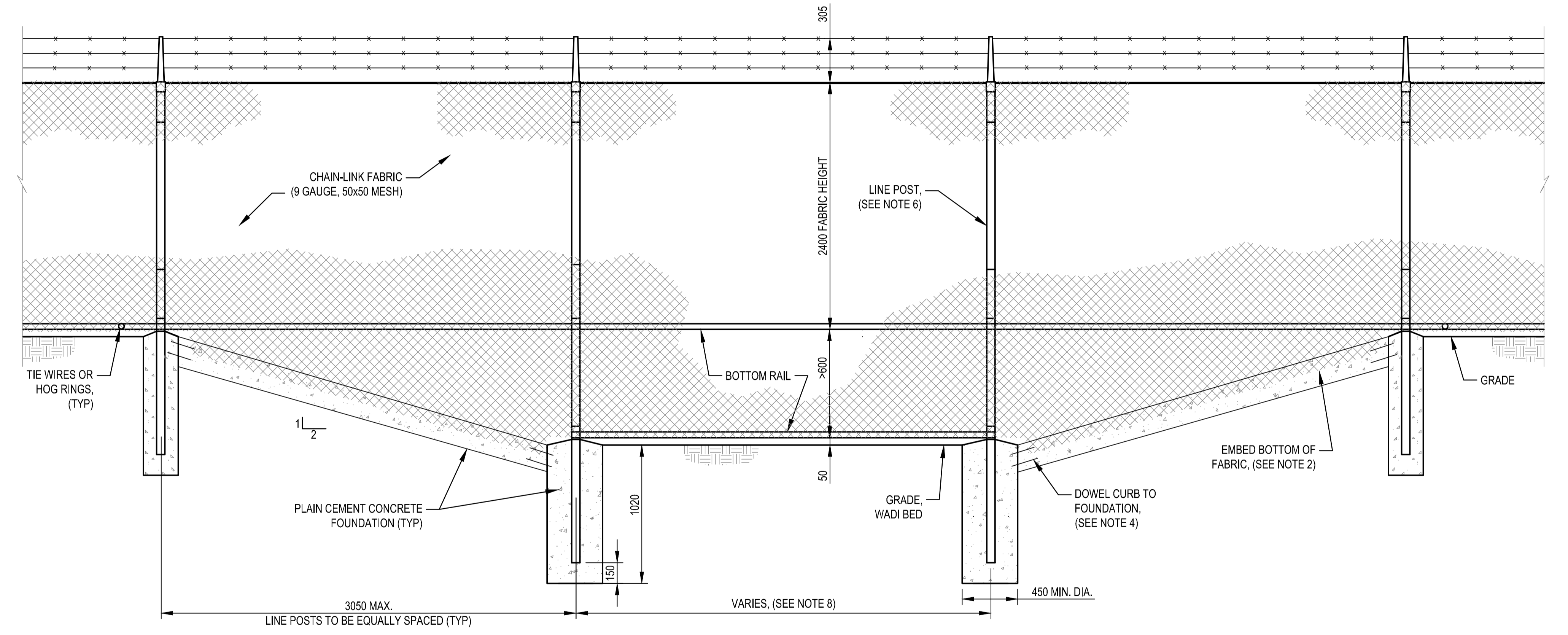
2 DETAIL - WADI CROSSING SCALE: NTS
